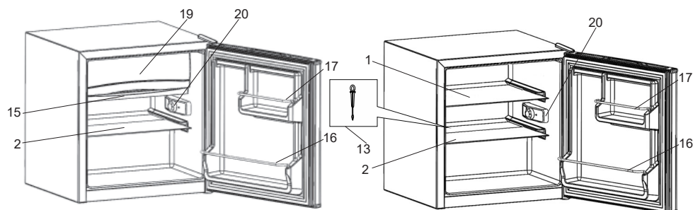
f) холодильники NSL 86, NSL 107
