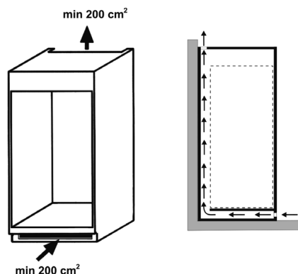
Рисунок Б.2 - Схема циркуляции воздуха вокруг холодильного прибора Сурет Б.2 - Тоңазытқыш прибор айналасындағы ауа айналысының схемасы
